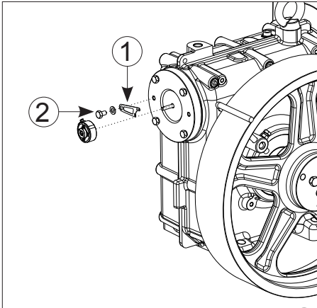
① شريحة التثبيت من Forcid ② برغي M10
