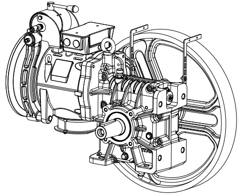
موتور بمجموعة تروس شاملا الملحقات التكميلية وفقا لمواصفات الطلبية
